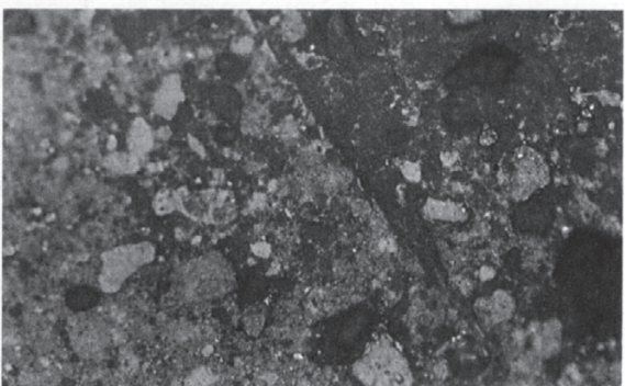
Fig. 11 Microscopio óptico, luz polarizada ampliación: x50, pasta III
