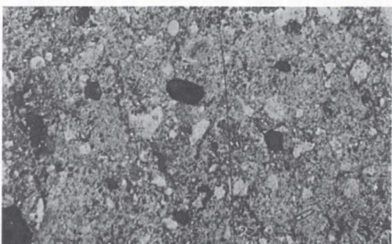
Fig. 8 Microscopio óptico, luz polarizada, ampliación: x50
