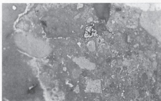
Fig. 4 Microscopio óptico, luz polarizada, amplificación x75
