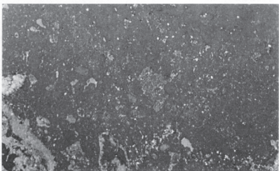
Fig. 10 Microscopio óptico, luz polarizada ampliación: x50, pasta II
