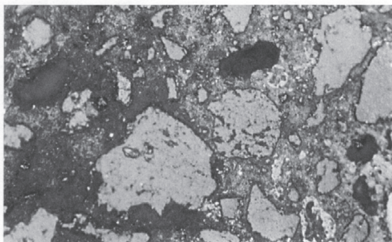
Fig. 9 Microscopio óptico, luz polarizada ampliación: x50, pasta I
